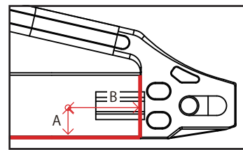
ネクスレイリアフェンダー 取付アダプター追加加工
