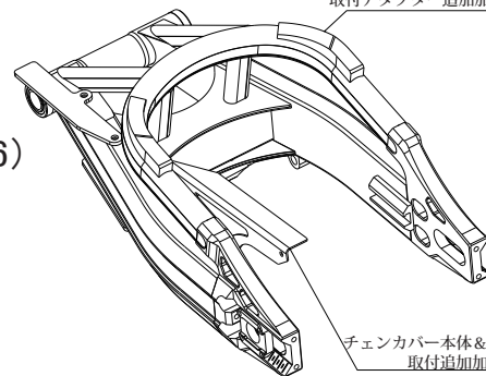
ネクスレイリアフェンダー 取付アダプター追加加工
